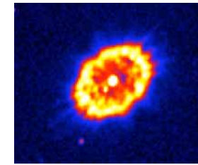
Nova Hercules (1934) DQ - Her
