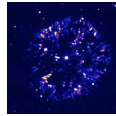
Nova Persei (1901) GK Per
