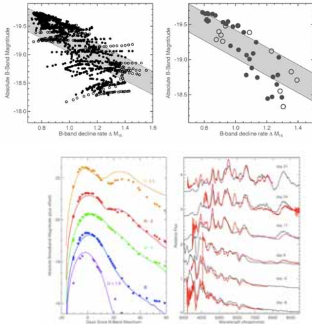
SN 2003 du vs Model
