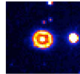
Nova Serpentis (1970) FH Ser
